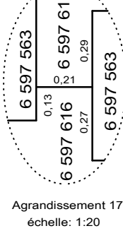
Agrandissement 17 échelle: 1:20
